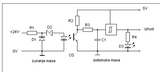
Električna shema vhodnega digitalnega modula za enosmerne napetosti
