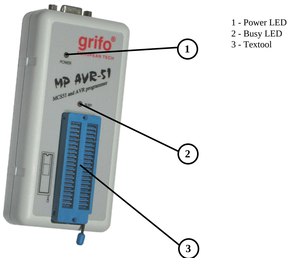
FIGURA 5: POSIZIONE LEDs E TEXTTOOL
