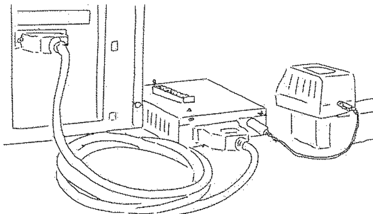
FIGURA 4: CONNETTORI DI ALIMENTAZIONE E PORTA PARALLELA
